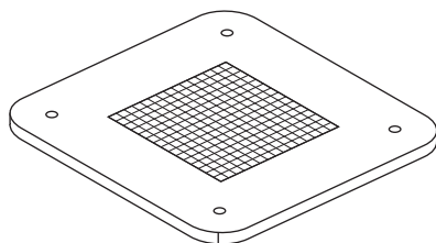
A 400*400*12mm(1pc)
